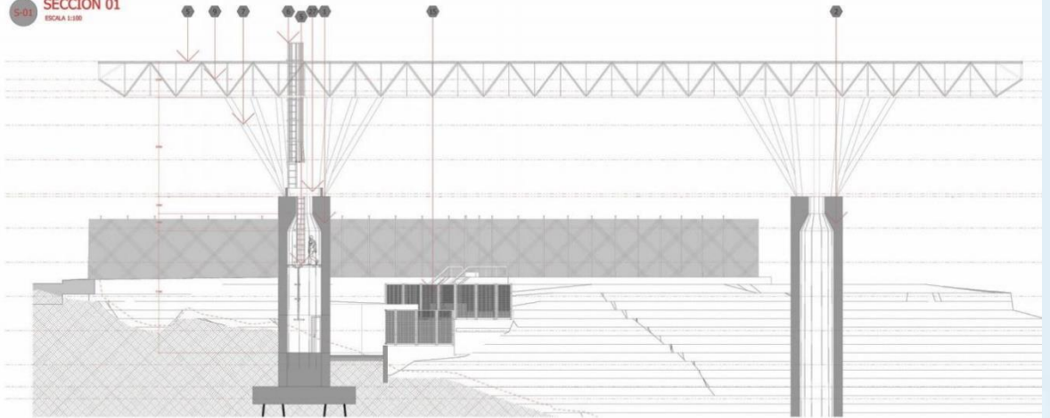
6-01 ALZADO NORTE ESCALA 1:100
